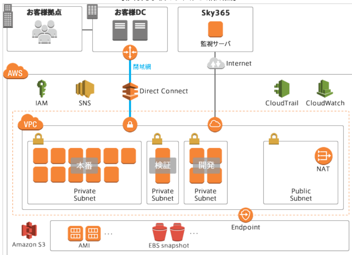
【移行完了後のシステム構成図】
